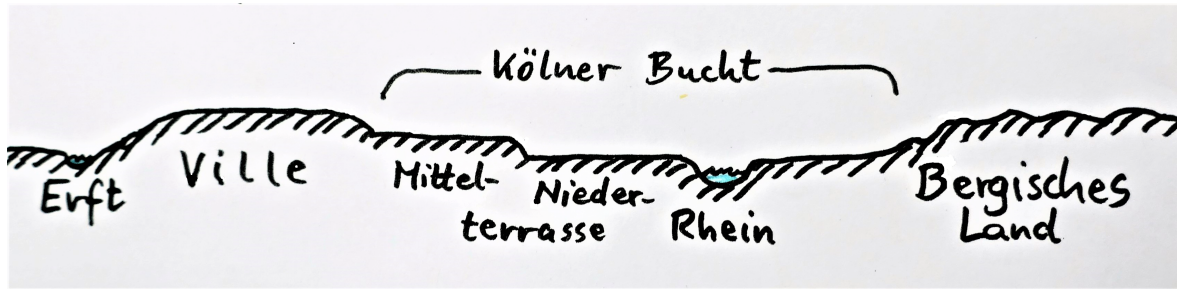
Das Landschaftsprofil der Kölner Bucht im Querschnitt, schematisch
